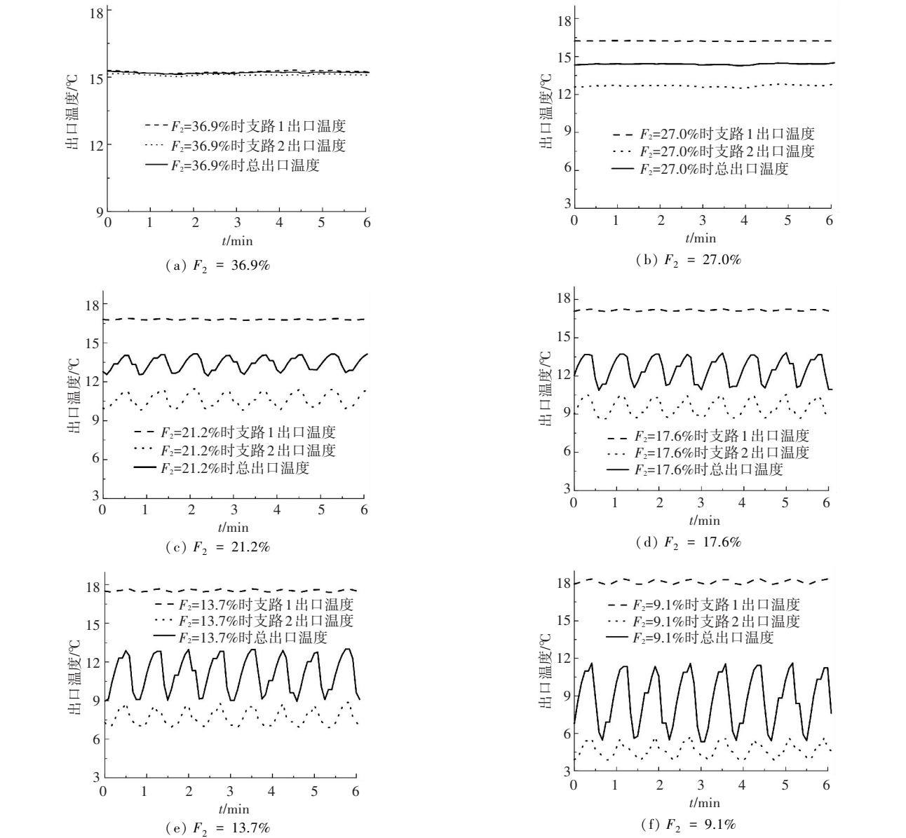
图 2 不同水流量下两支路及总出口温度随时间的变化
