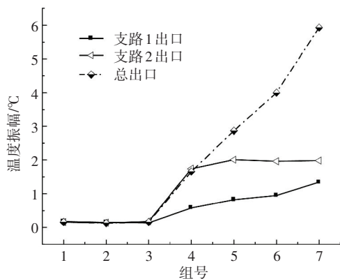
图 3 两支路及总出口的温度振幅随水流量非均匀率的变化
