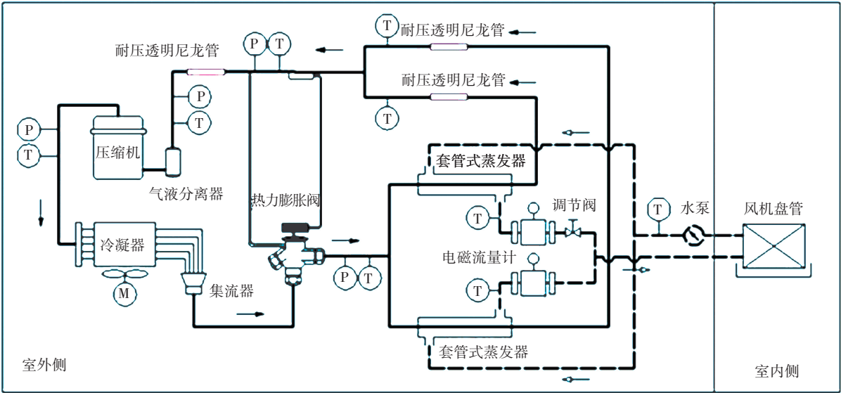
图 1 实验台系统流程
