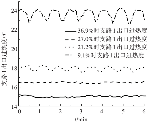
图 5 不同水流量非均匀率下支路 1 出口过热度
