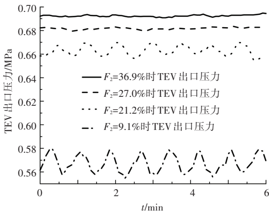
图 7 不同水流量非均匀率下 TEV 出口压力
