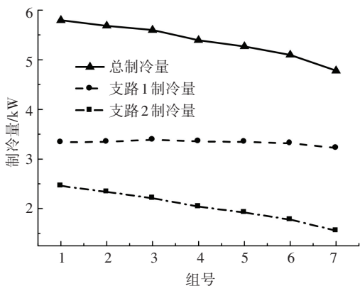
图 6 蒸发器制冷量随水流量非均匀率的变化
